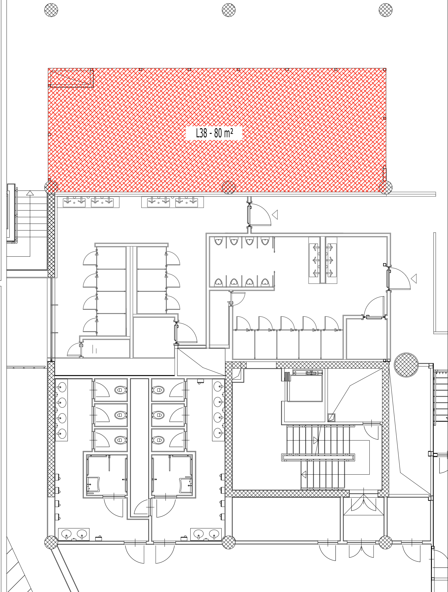
PLANIMETRIA DI DETTAGLIO Scala 1/100
